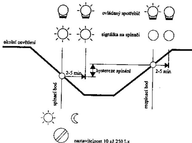
obr. 3 Časový diagram spínání
